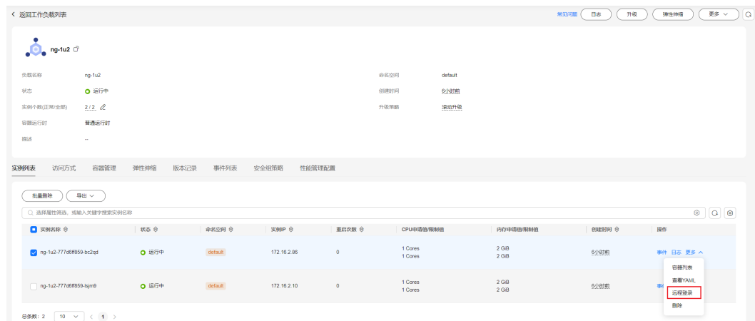
图 2-12 登录容器
