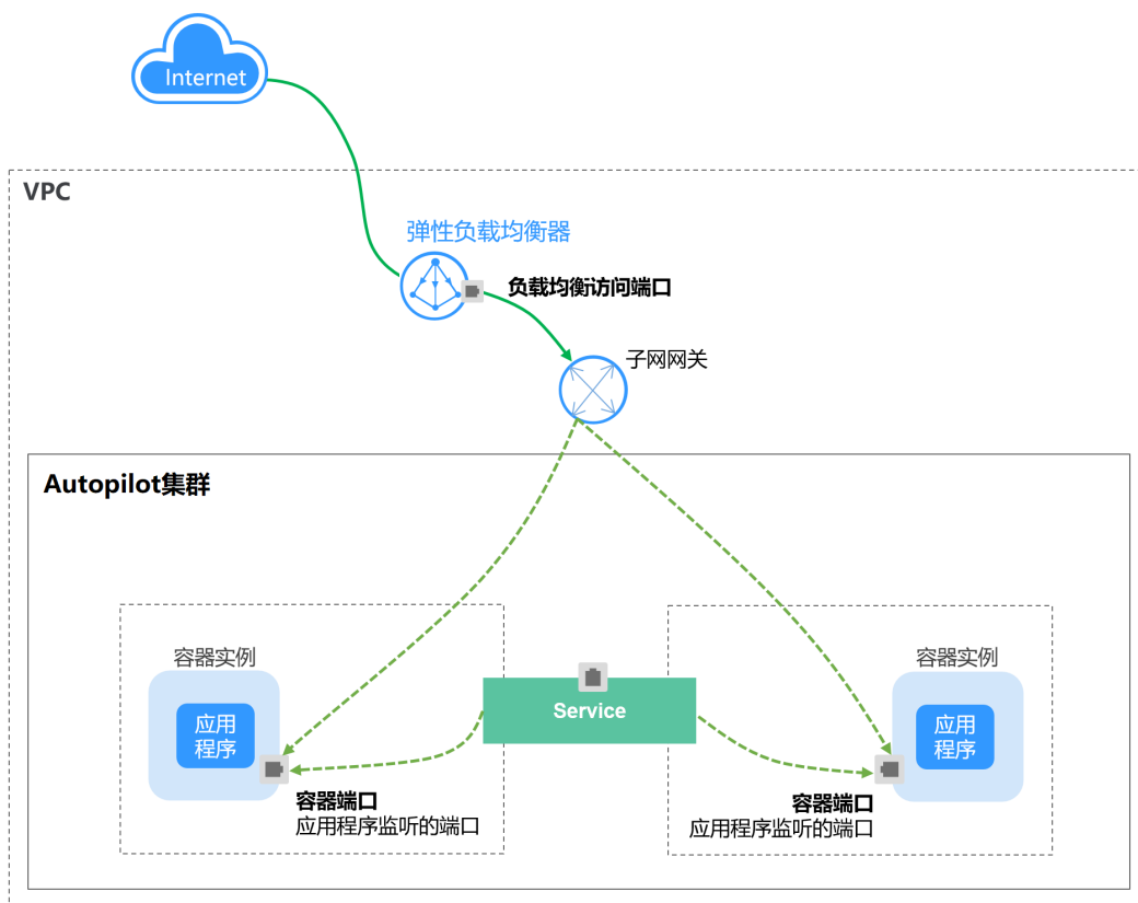
图 3-5 ELB 直通容器
