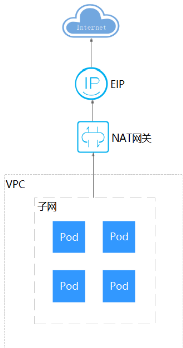
图 3-11 SNAT
