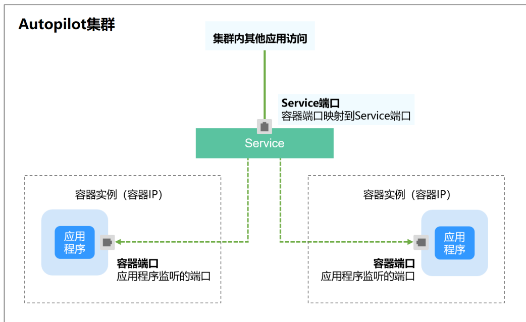
图 3-4 集群内访问
